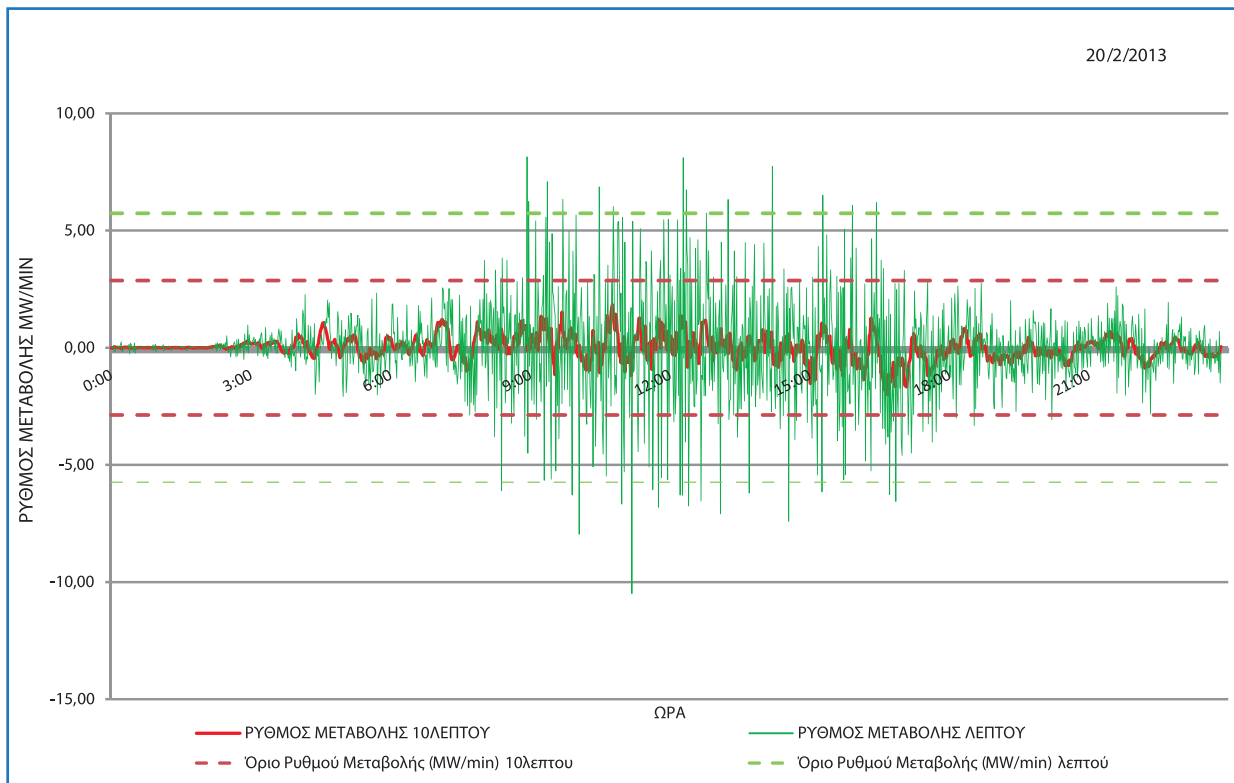
Σχ. 8 - Ρυθμός Μεταβολής Αιολικής Ηλεκτροπαραγωγής
