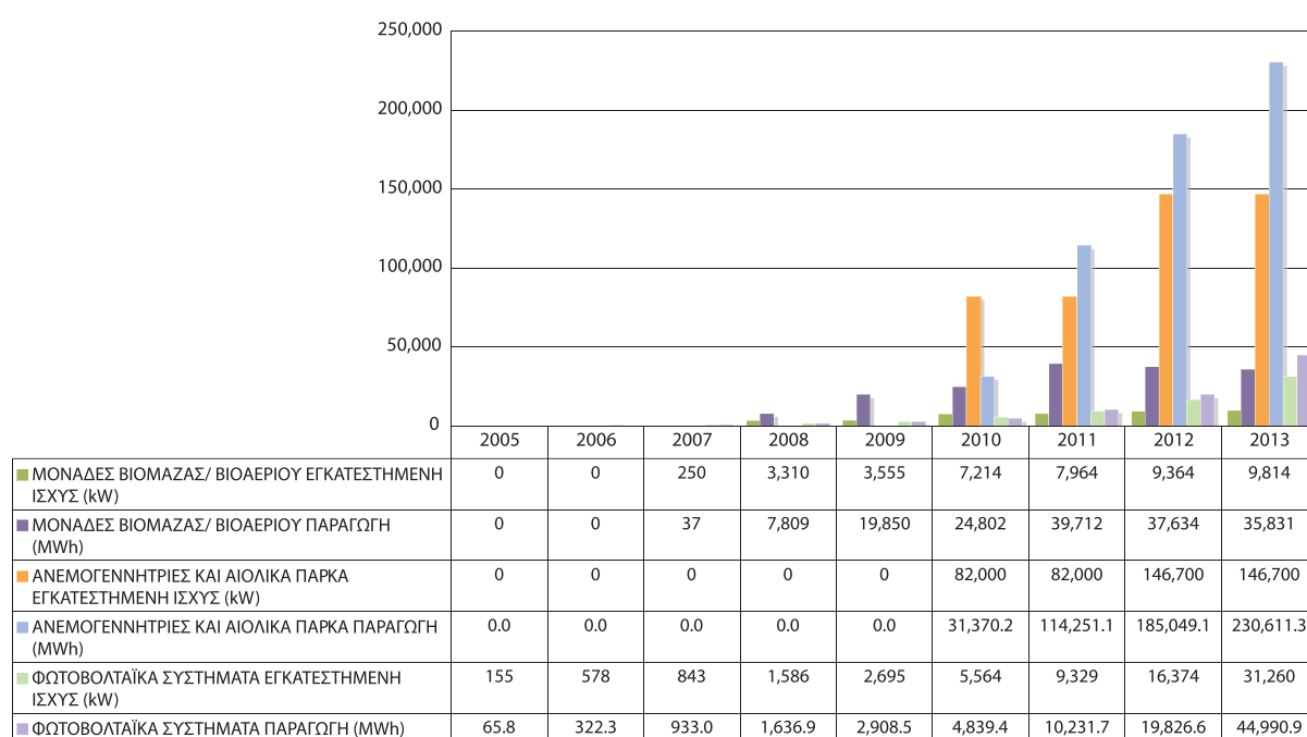
Γραφική Παράσταση 4- Ετήσια εγκατεστημένη Ισχύς (kW)/ Παραγωγή (MWh) ΑΠΕ
