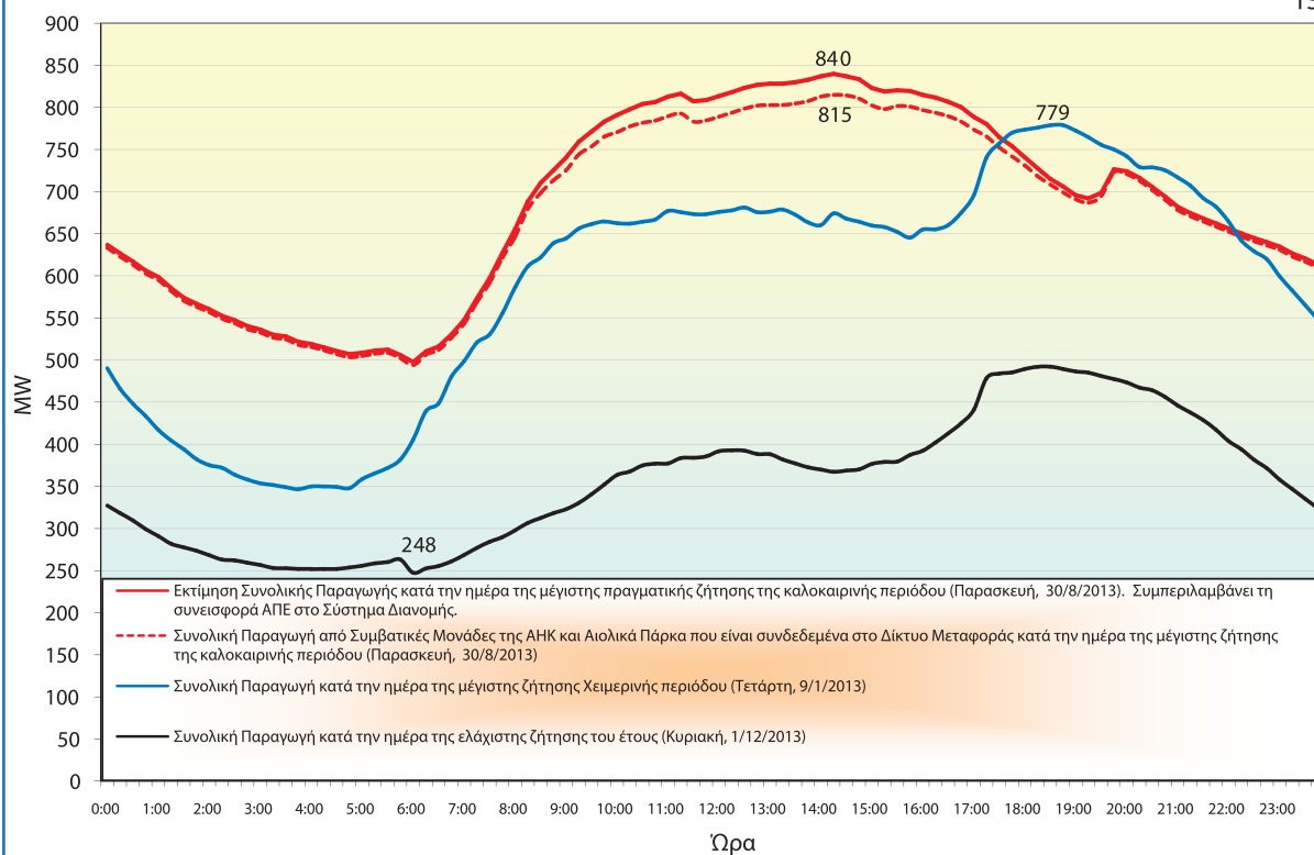
Σχ. 16 - Ημερήσια Διακύμανση στη Συνολική Παραγωγή κατά τις Ημέρες της Μέγιστης και Ελάχιστης Ζήτησης του Έτους 2013
